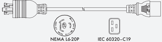
NEMA L6-20P
