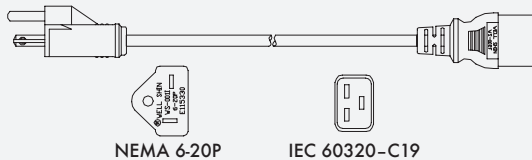
NEMA 6-20P
